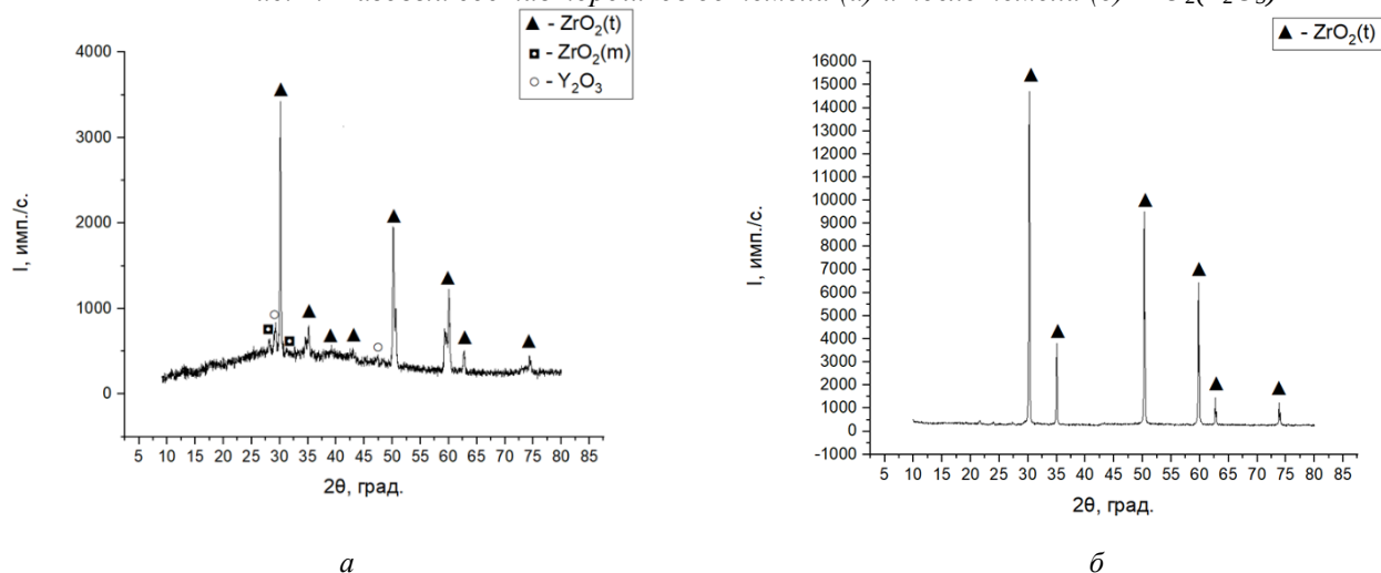
Рис. 3. Фазовый состав спечённых порошков без помола (а) и с помолом (б) \text{ZrO}_2(\text{Y}_2\text{O}_3)
