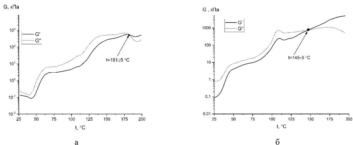
Рисунок 2. Изменение модуля упругости G' , модуля потерь G'' клеевых композиций от температуры (а) с дисперсной фазой корунда и (б) с добавкой Al(OH)_3
