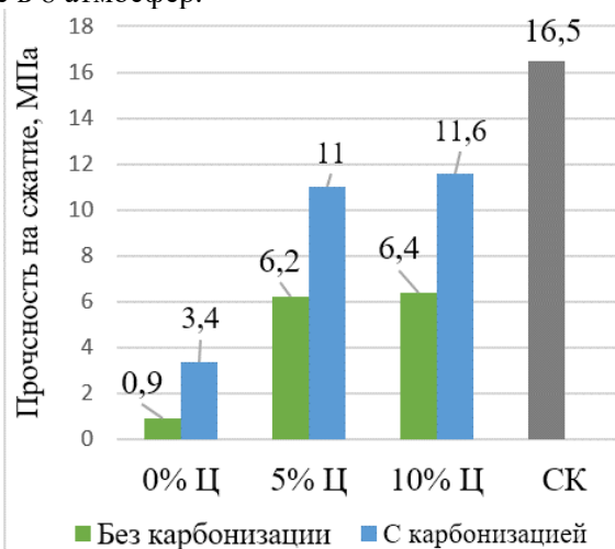
Рис.3 – Прочность на сжатие исследуемых карбонизированных составов на 1 сутки (а) и на 28 суток (б)
