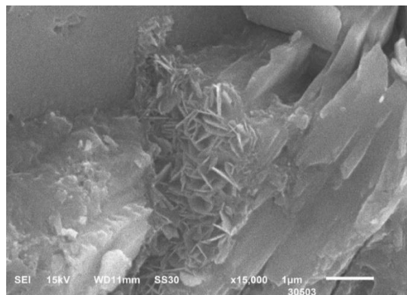
Рис. 5. Микрофотография цемента с т/а глиной 650С: увеличение: а – \times 5\,000 ; б – \times 15\,000 .
