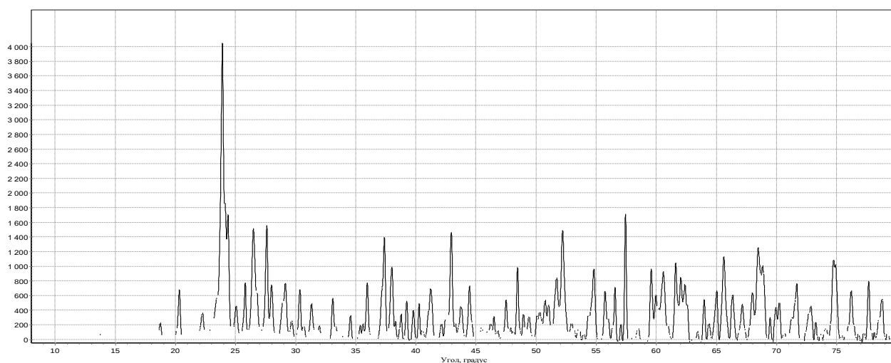
Рис. 2. Дифрактограмма бентонитфосфатной связки, обожженной при 900 °C
