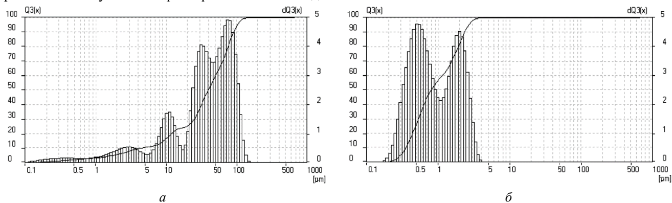
Рис. 1. Гранулометрический состав термообработанных порошков \text{ZrO}_2(\text{Y}_2\text{O}_3) до (а) и после (б) измельчения
