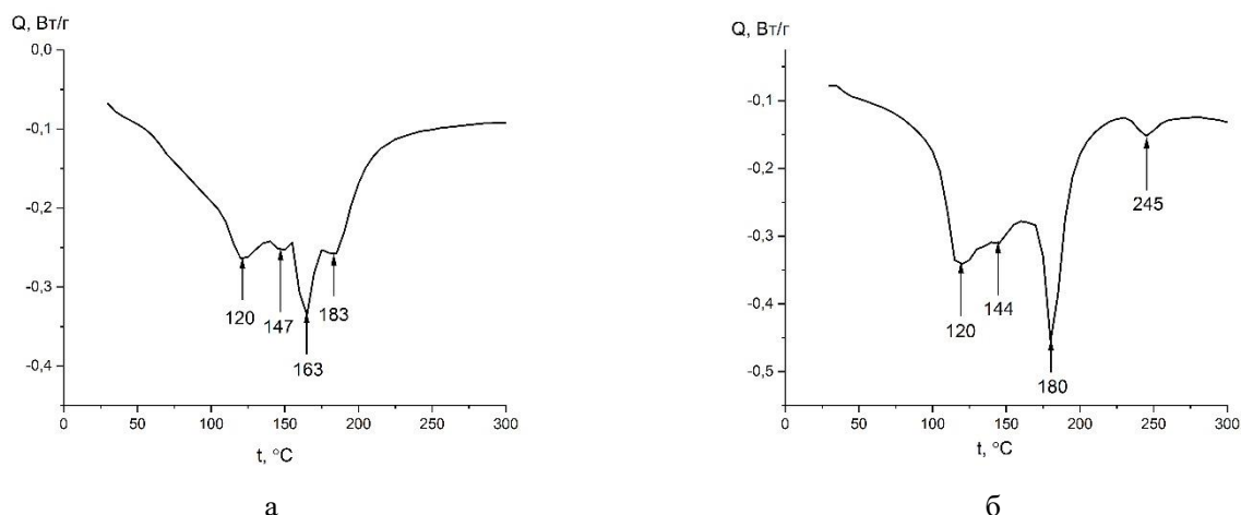
Рисунок 3. Кривые ДСК клеевых композиций от температуры (а) с дисперсной фазой корунда и (б) с добавкой Al(OH)_3
