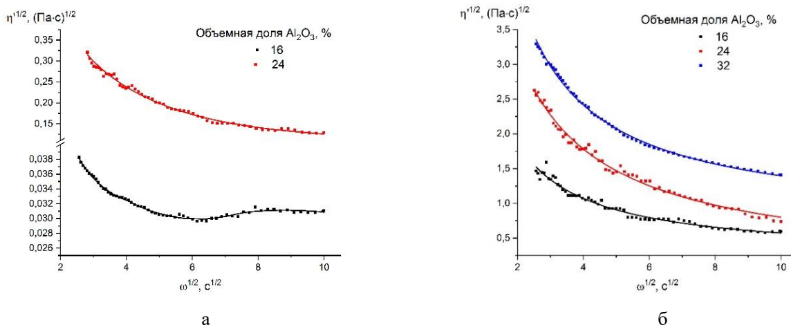
Рисунок 1. Частотные зависимости вязкости композиций на основе (а) АФС и (б) АХФС с дисперсной фазой корунда
