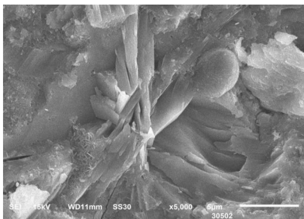
Рис. 5. Микрофотография цемента с т/а глиной 650С: увеличение: а – \times 5\,000 ; б – \times 15\,000 .
