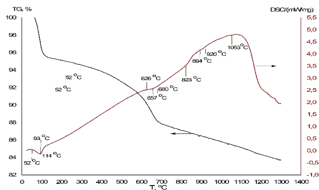
Рис. 1. ТГ/ДСК кривые бентонита; скорость нагрева 5 °C/мин
