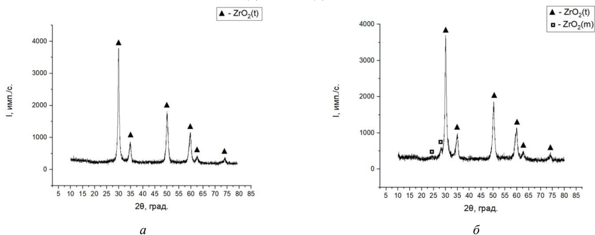
Рис. 2. Фазовый состав порошков до помола (а) и после помола (б) \text{ZrO}_2(\text{Y}_2\text{O}_3)
