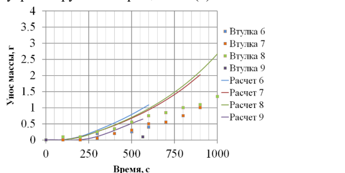
Рисунок 5 – Расчетный и экспериментальный унос массы для втулок 6 - 9.
