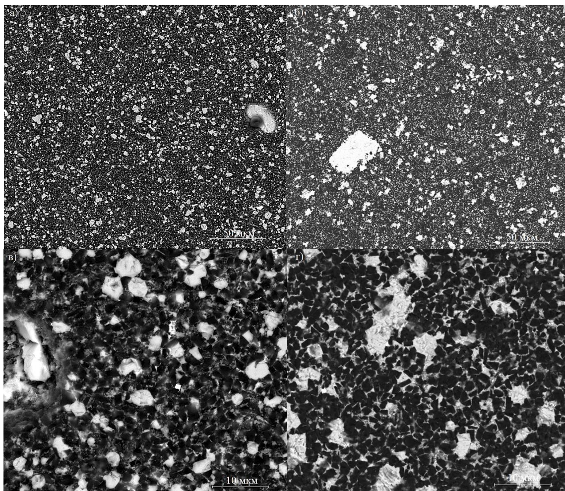
Рис. 1. Микроструктура экспериментальных изделий на основе cBN: (а, в) – образец 1; (б, з) – образец 2. Увеличение (а, б) – 500 × , (в, з) – 2500 ×
