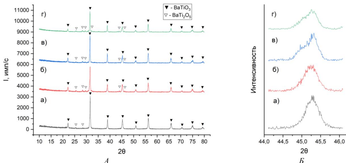
Рис. 2. Фазовый состав порошков (А) и дифракционный рефлекс \text{BaTiO}_3 (Б), синтез при температуре: а) 800 °С, б) 1000 °С, в) 1200 °С, г) 1300 °С.
