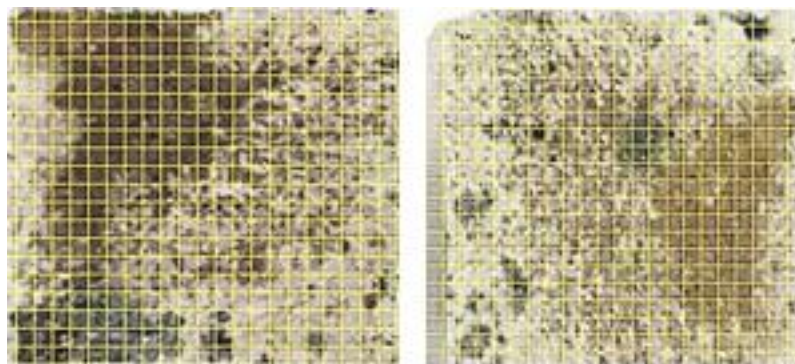
Рис.1 – Глубина карбонизации при различных давлениях прессования 100 кгс/см 2 (а) и 300 кгс/см 2 (б)
