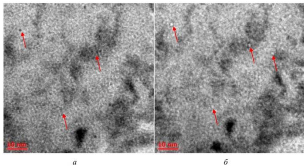
Рисунок – ПЭМ-изображения в режиме высокого разрешения структуры облученного образца Zr(Nb)N (300 снэ; расстояние от поверхности \sim 1\,250 - 1\,320 нм).
