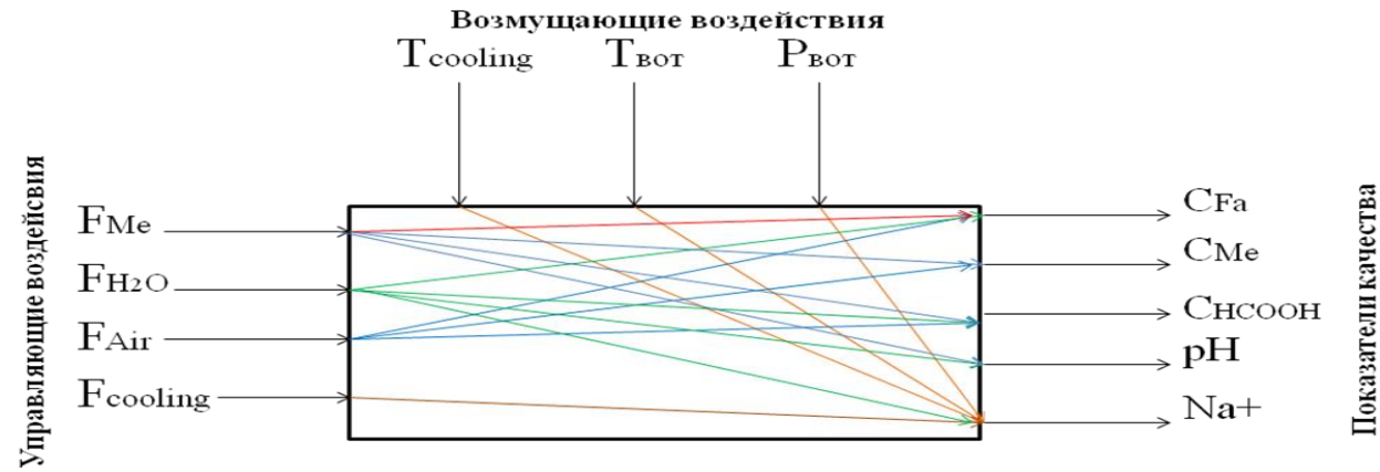
Рис. 1. Структурная схема производства формалина, как объекта управления качеством:
